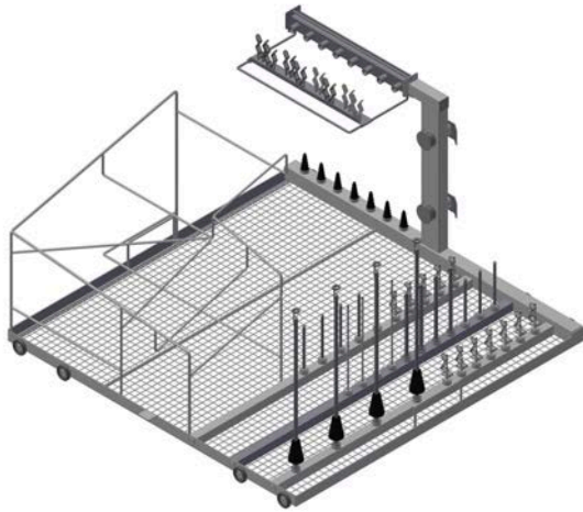
Anestesia- ja kirurgian pesuteline
